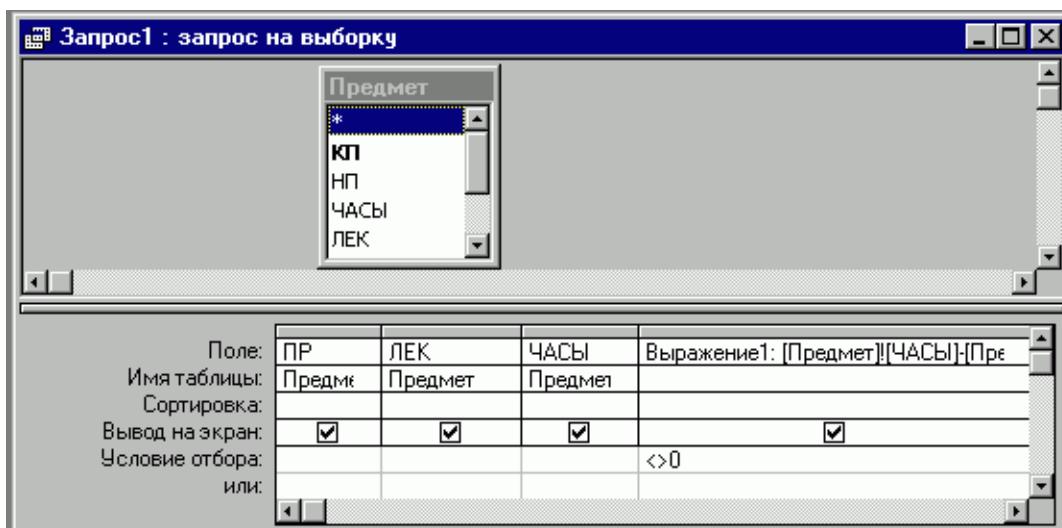
Рисунок 127. Окно запроса с вычисляемым полем
