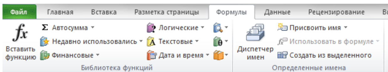
Рисунок 80. Панель «Формулы»
