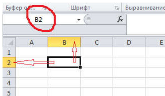
Рисунок 69. Адрес ячейки
