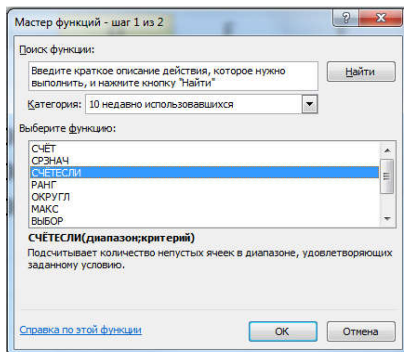
Рисунок 83. Выбор функции
