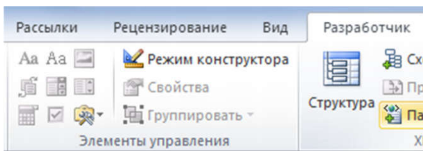
Рисунок 57. Вкладка Разработчик
