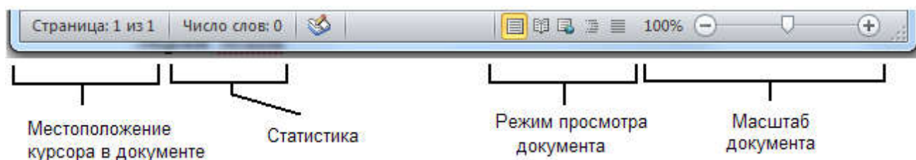
Рисунок 2. Строка состояния
