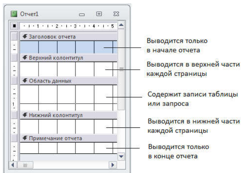
Рисунок 133. Разделы отчета
