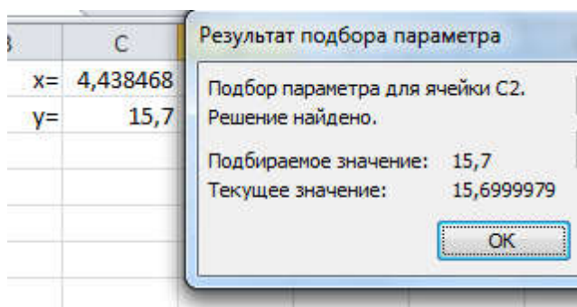
Рисунок 114. Найденный результат
