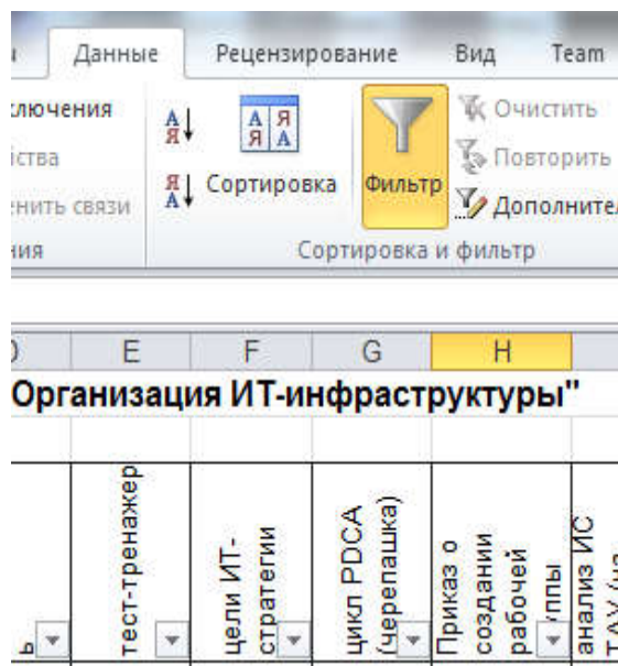
Рисунок 104. Отражение автофильтра
