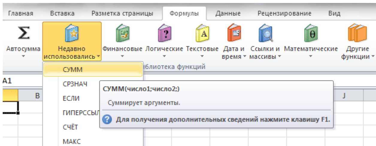
Рисунок 81. Выбор функции
