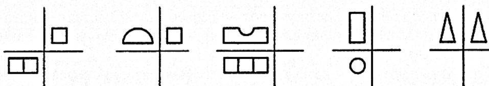
а) Незавершенные схемы-развертки отдельных деталей.
